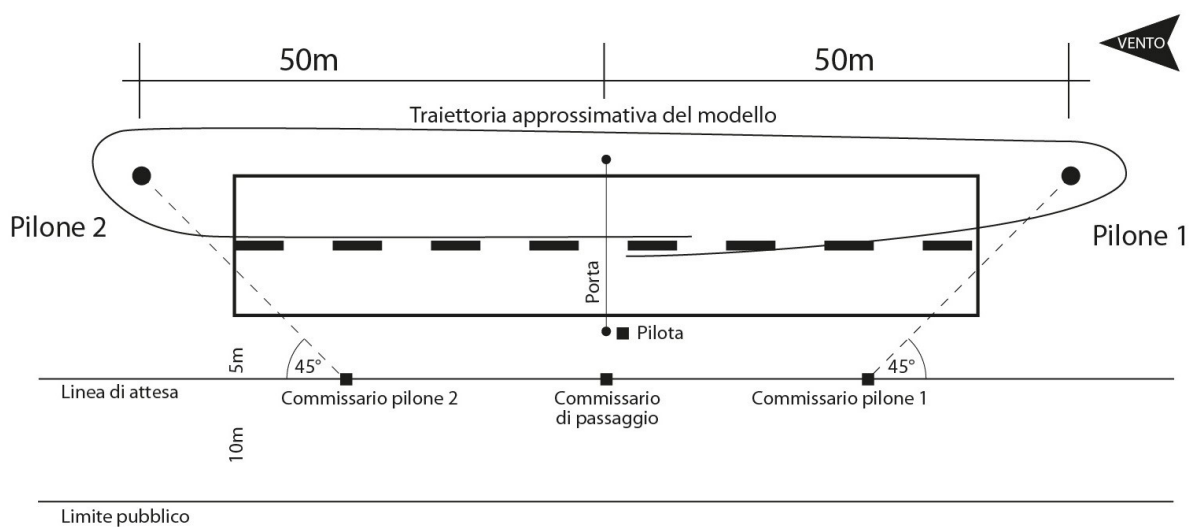
Fig. 1 – Planimetria campo di gara LMBO FANI
